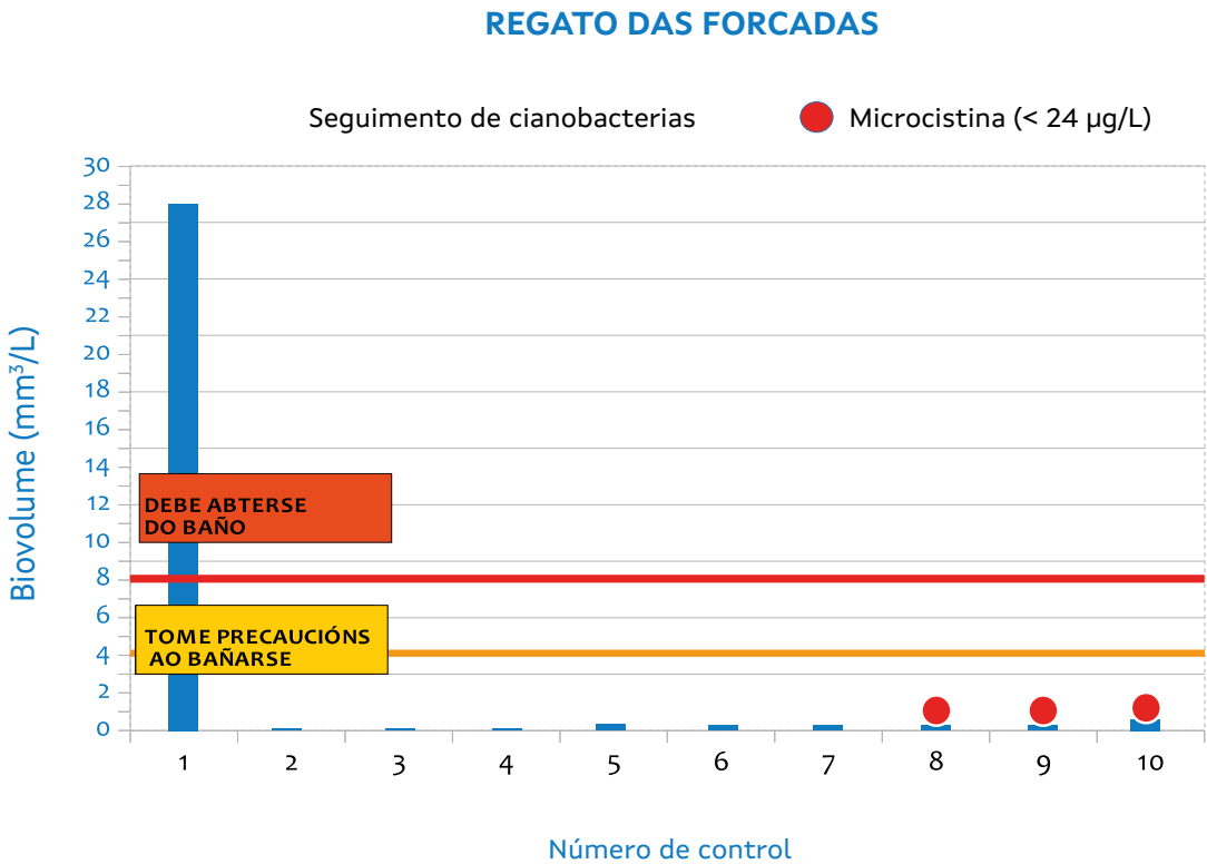
Figura 9. Seguimento de cianobacterias no regato das Forcadas na tempada 2024
