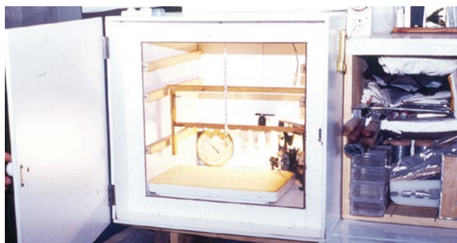
Diferentes incubadoras apícolas artesanais
