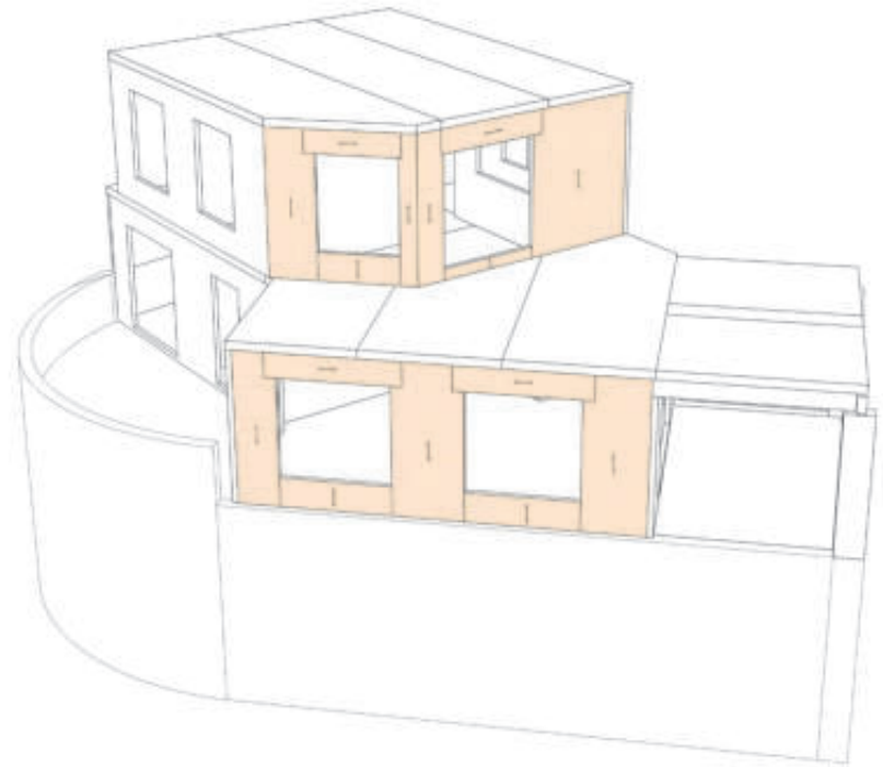
Esquemas estructurales en 3D © ESCUADRÍA
