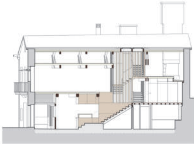
Sección
