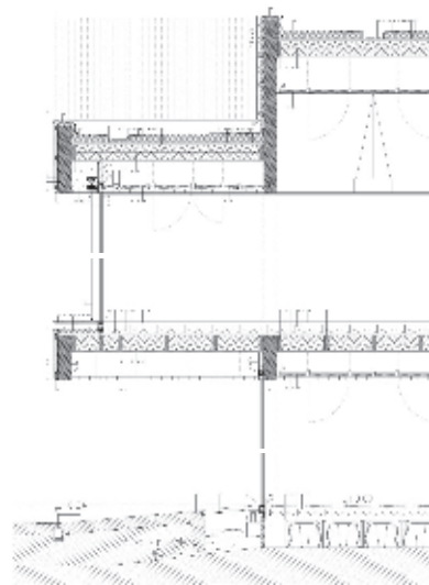
Sección constructiva
