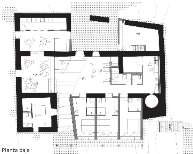
Planta baja
