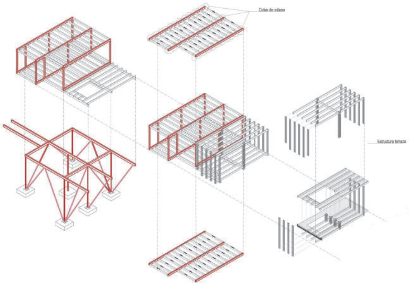
Estructura módulo de cabaña
