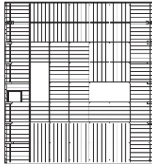
Esquemas estructurales en planta (forjados de pl. primera y cubierta)
