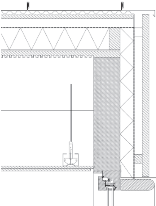
Sección constructiva vertical (envolvente-hueco)
