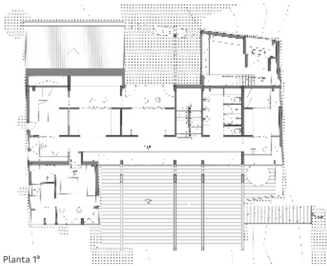
Planta 1º
