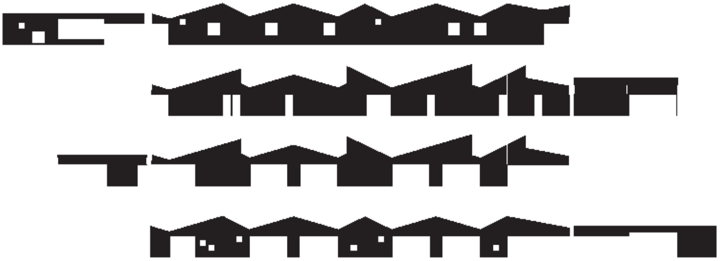
Alzados de muros de madera contralaminada
