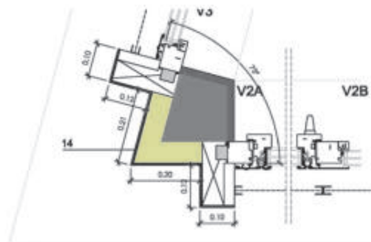
Detalles de cerramiento, huecos y carpinterías
