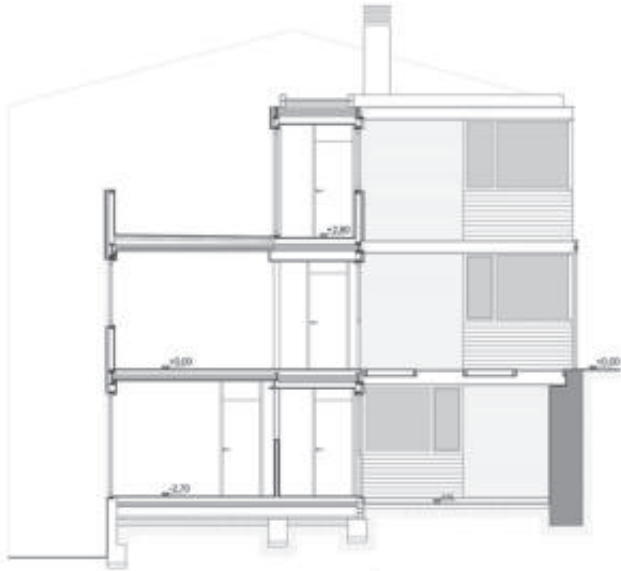
Sección
