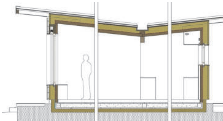
Sección
