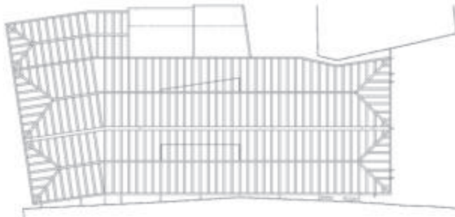
Esquema estructural de cubierta (planta)
