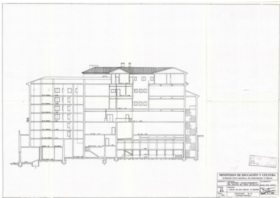
Plano transversal do ARG. Reforma de 2003 / Ministerio de Educación e Cultura. Madrid, 2003. En: Expediente de reforma do edificio do ARG. Arquivo de xestión do ARG [Sen signatura: no despacho de dirección].
