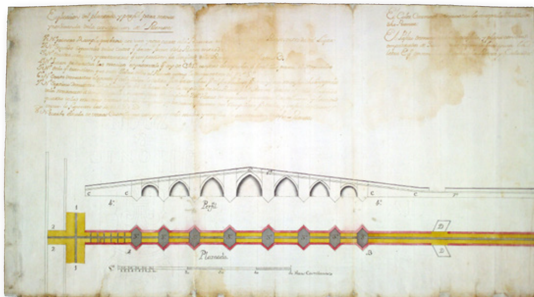
Perfil e planta da ponte de Cedeira.- Escala [ca. 1:229] 50 varas castelás [=18,2 cm].- [Cedeira: s.n., 1764] 1 p.: ms, tt, ag, col; 32x56 cm Extraído de: Informe enviado polo intendente xeral de Galicia ao Real e Supremo Consello de Castela sobre a construción da ponte da vila de Cedeira. 1764. Sig. 46537/3 ARG. Colección cartográfica e iconográfica. CC.RI. 002
